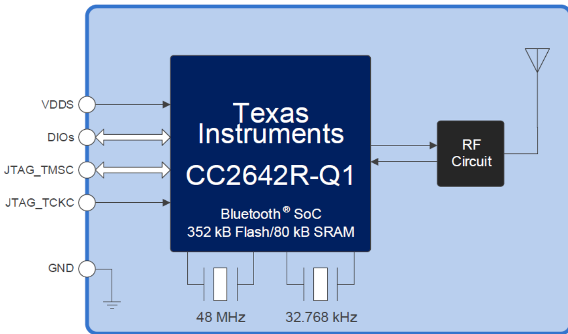
HRM3012ブロック図
