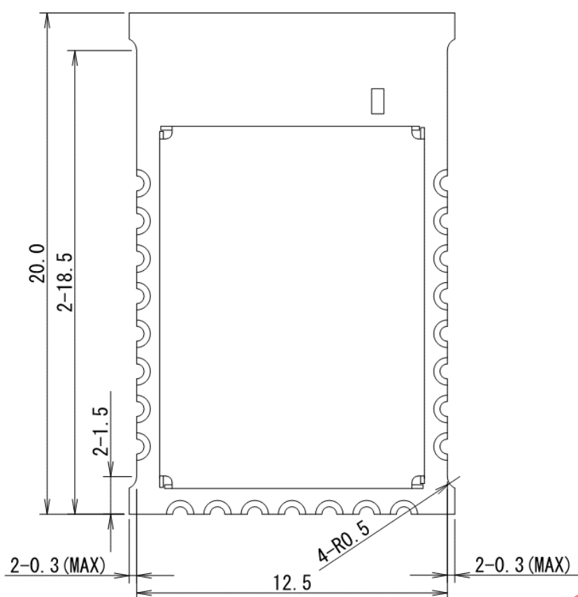
<Top View / Top 面視>
