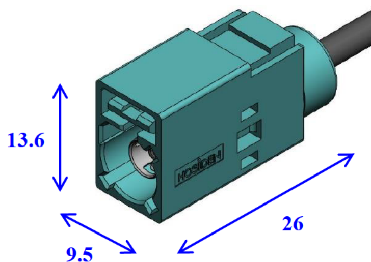
嵌合図
