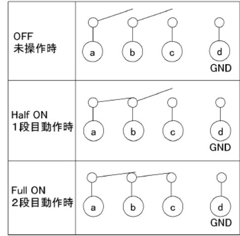
Circuit Diagram 回路図
